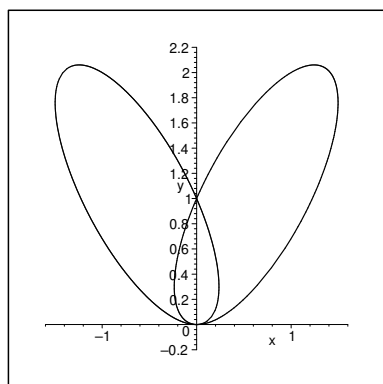
Fig. 4.3.3 tacnode
