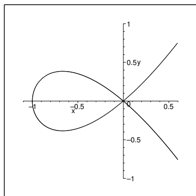
Fig. 4.3.1 parametric cubic
